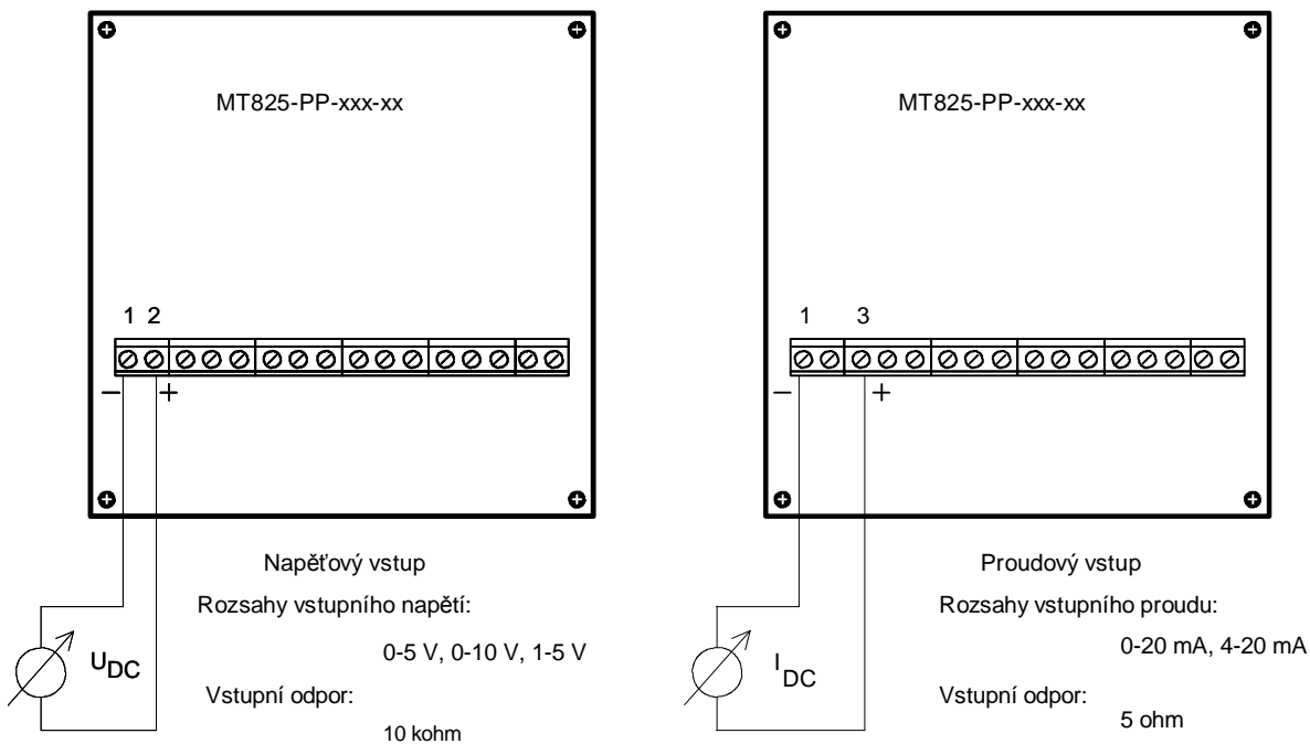
Obr.6 Zapojení napěťových a proudových procesových vstupů
