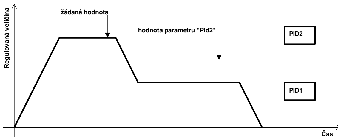
Obr.14 Dvě sady PID parametrů
